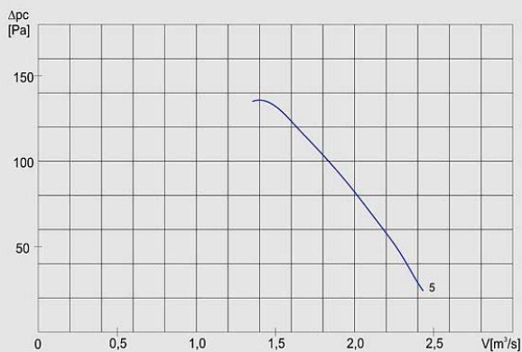
Charakterystyka aerodynamiczna WOJM-50
