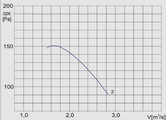
Charakterystyka aerodynamiczna WOJK-56
