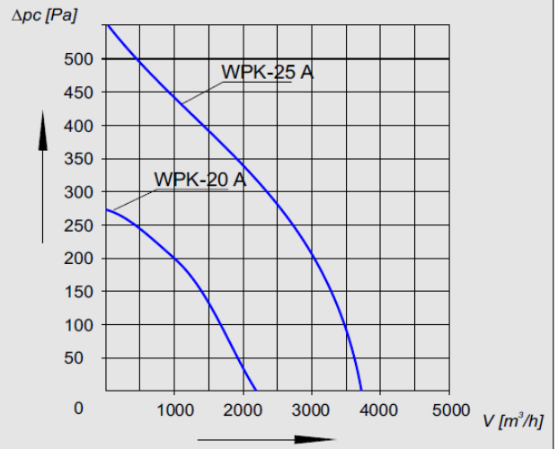
Charakterystyka aerodynamiczna WPK-20,25
