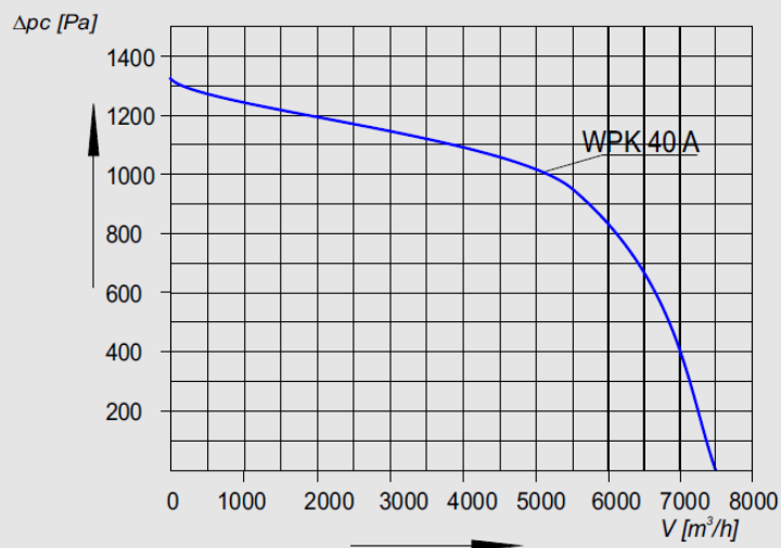
Charakterystyka aerodynamiczna WPK-40 A
