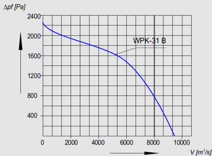
Charakterystyka aerodynamiczna WPK-31B
