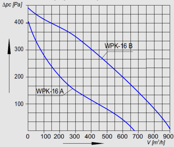
Charakterystyka aerodynamiczna WPK-16
