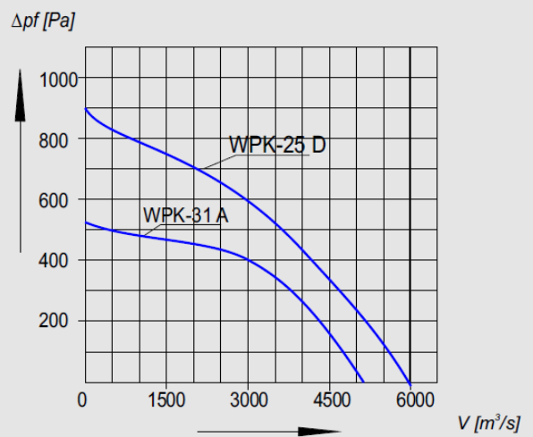
Charakterystyka aerodynamiczna WPK-25D, WPK-31A
