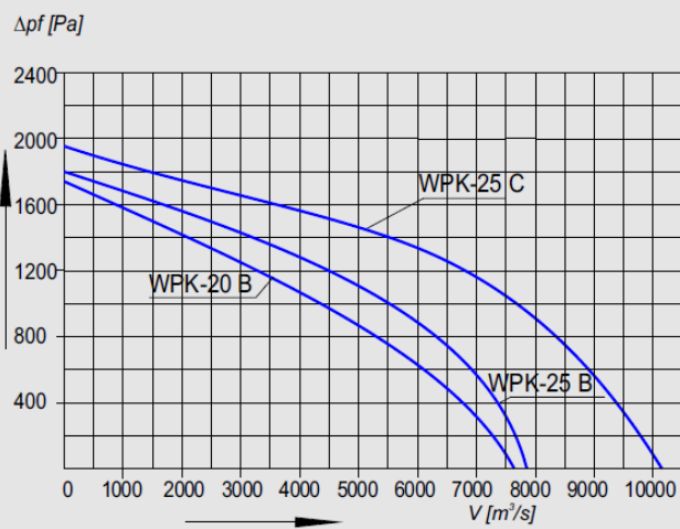
Charakterystyka aerodynamiczna WPK-20, 25
