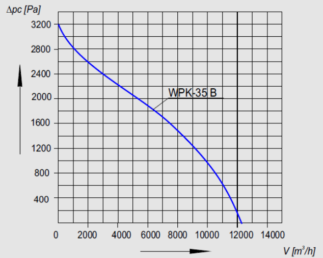
Charakterystyka aerodynamiczna WPK-35 B
