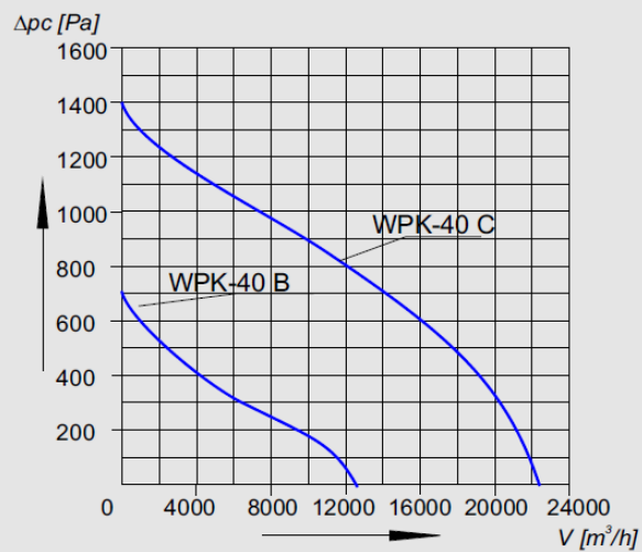
Charakterystyka aerodynamiczna "WPK-40"
