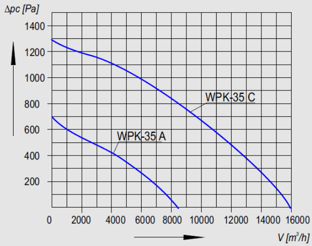
Charakterystyka aerodynamiczna WPK-35
